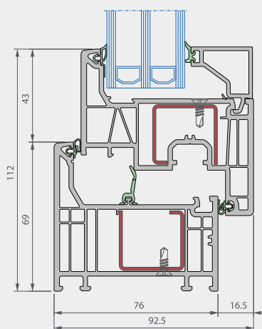
Przekrój pionowy
